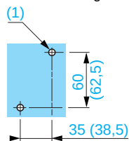
(1) 2 x M4 or 2 x Ø4.5
